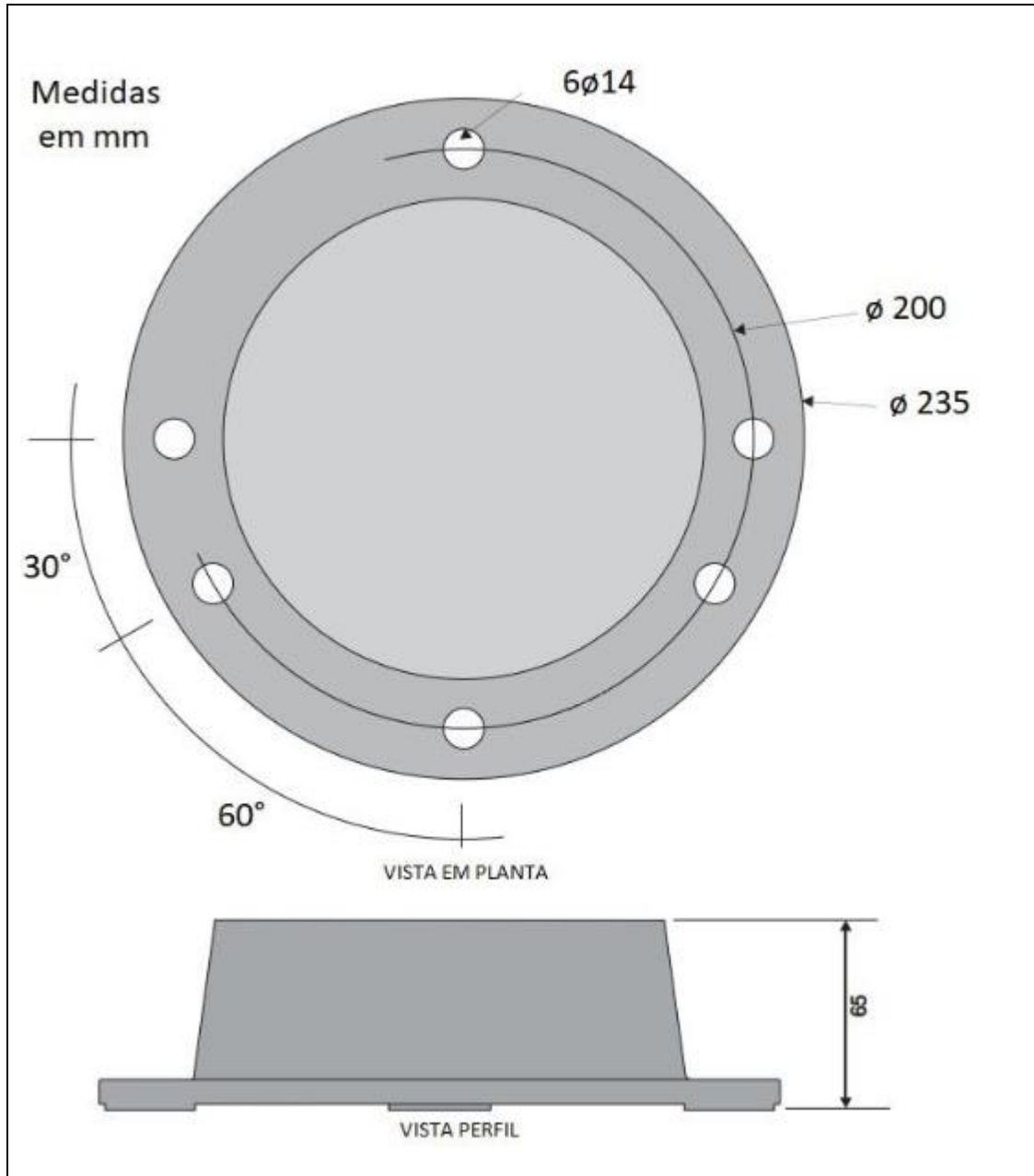
Figura 01: Tipo da furação da base da lanterna Verde 5/6MN;
