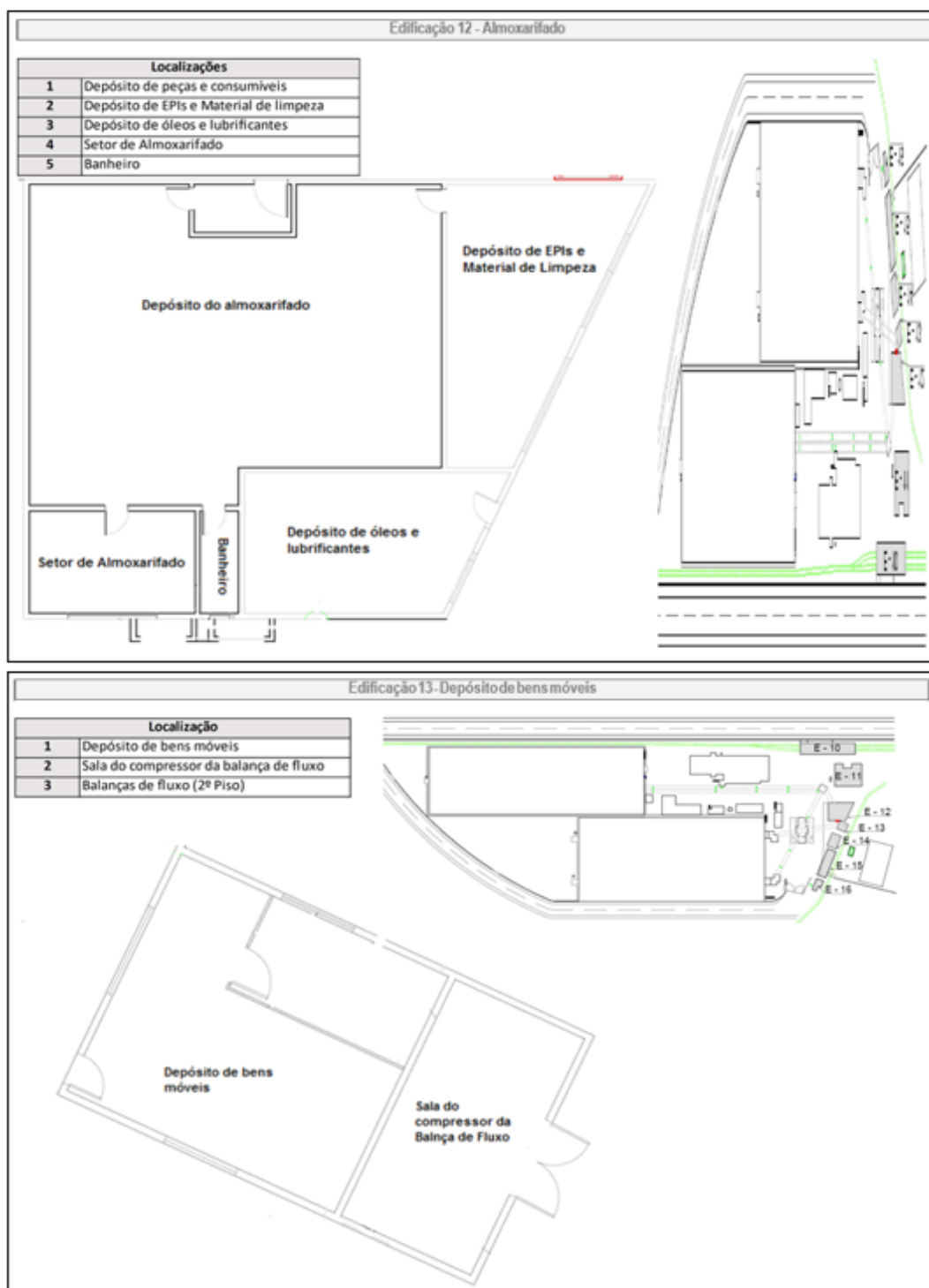
Figura 10 – Almojarifado e depósito de bens móveis.
