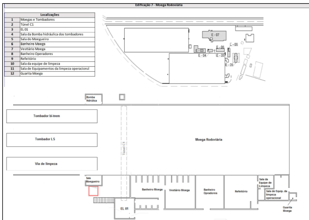
Figura 7 – Moega Rodoviária.
