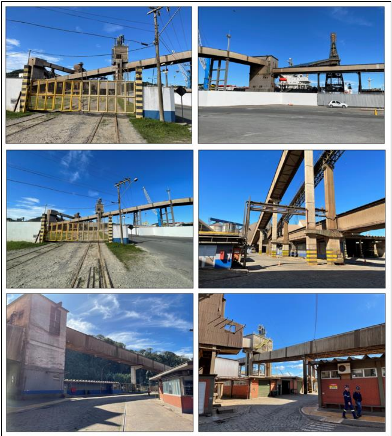
Figura 12 – Galerias de estrutura metálica.
