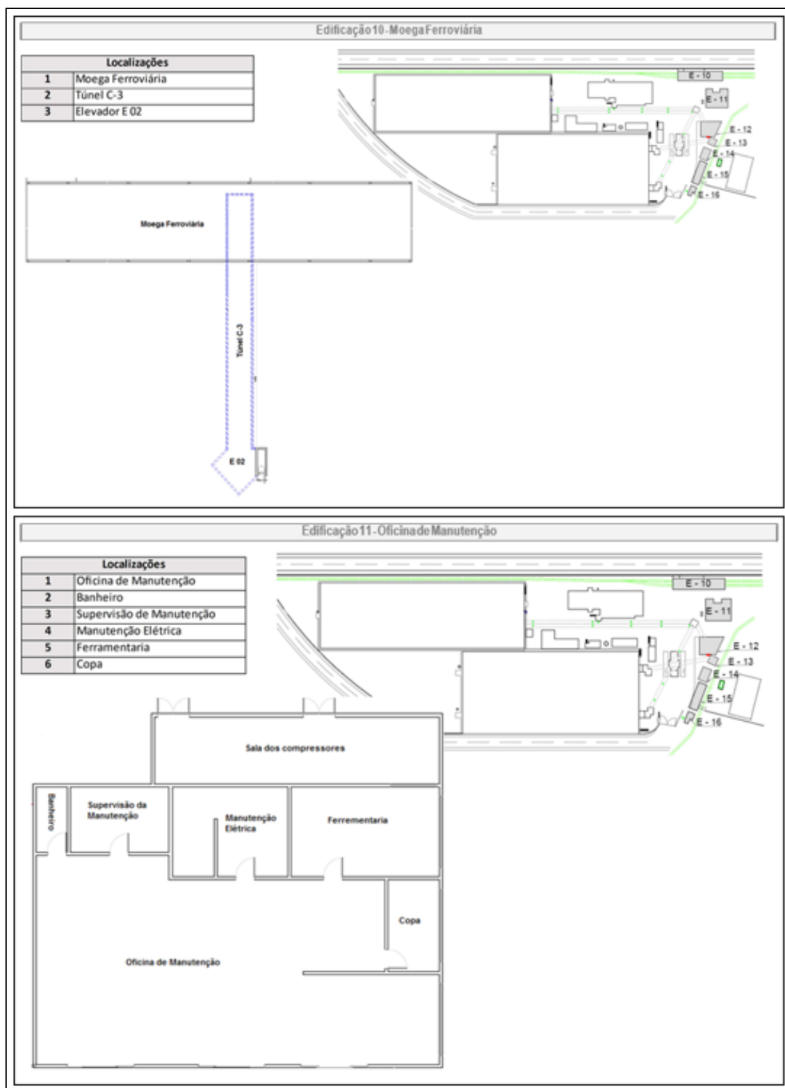
Figura 9 – Moega ferroviária e oficina de manutenção.
