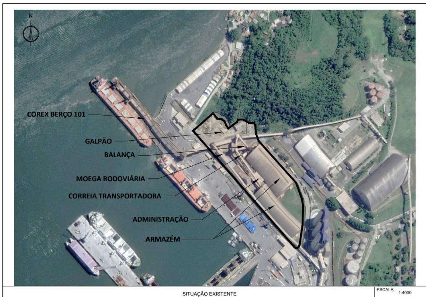
Figura 1 – Situação existente do terminal. Fonte: NCA Engenharia, Arquitetura e Meio Ambiente.
