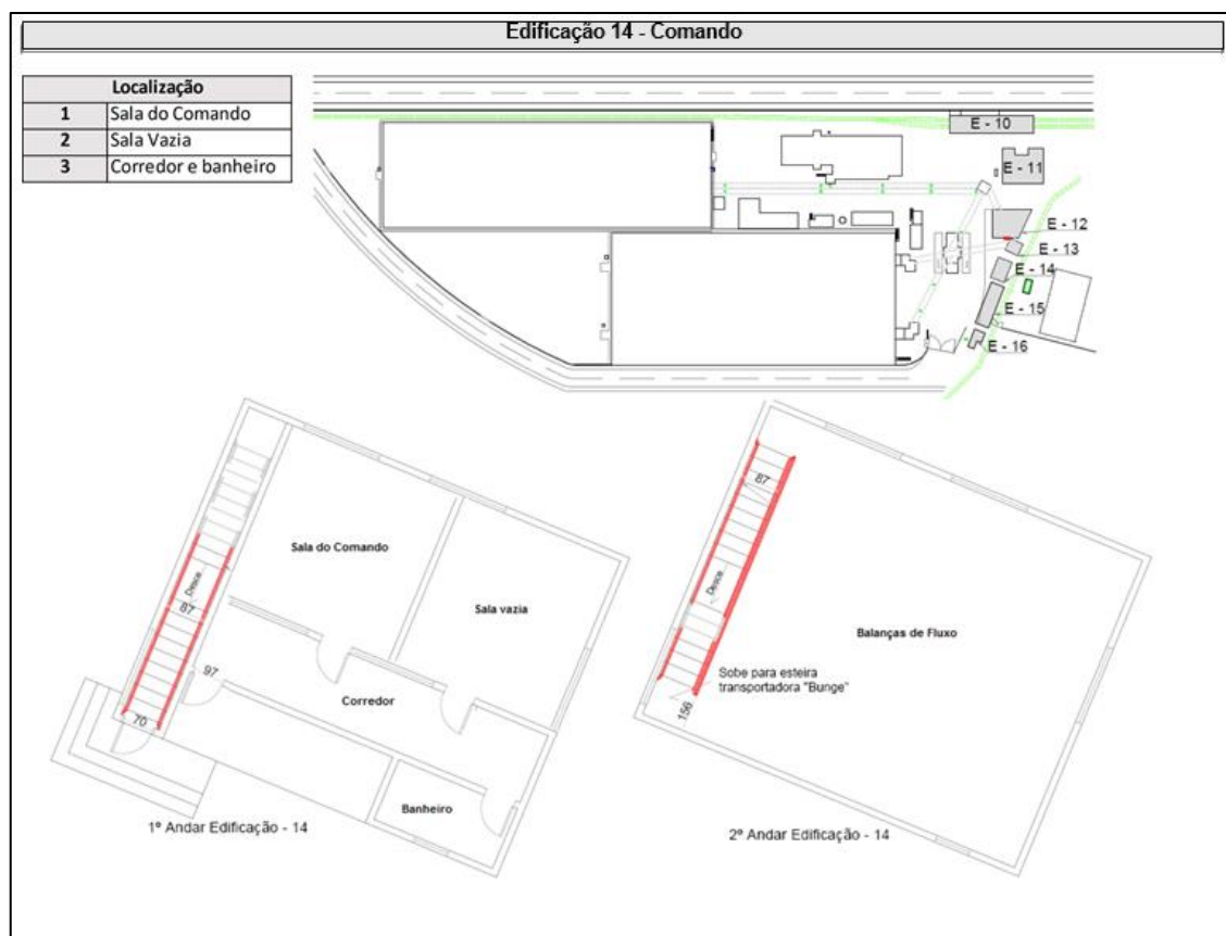
Figura 11 – Comando.
