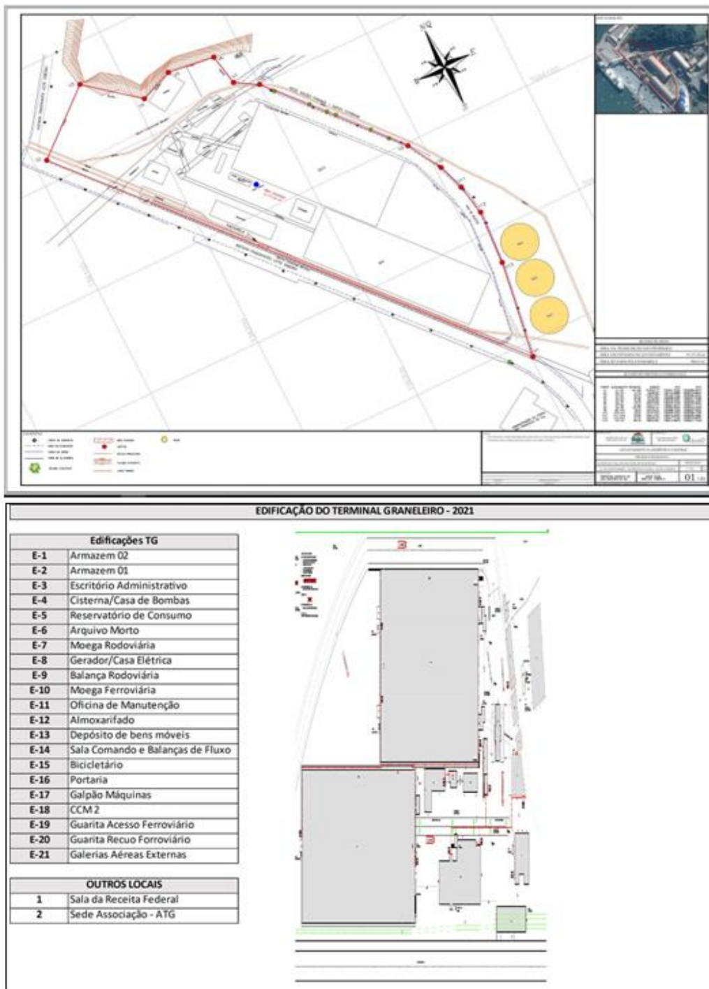
Figura 3 – Delimitação da área, planta e edificações do TGSFS.
