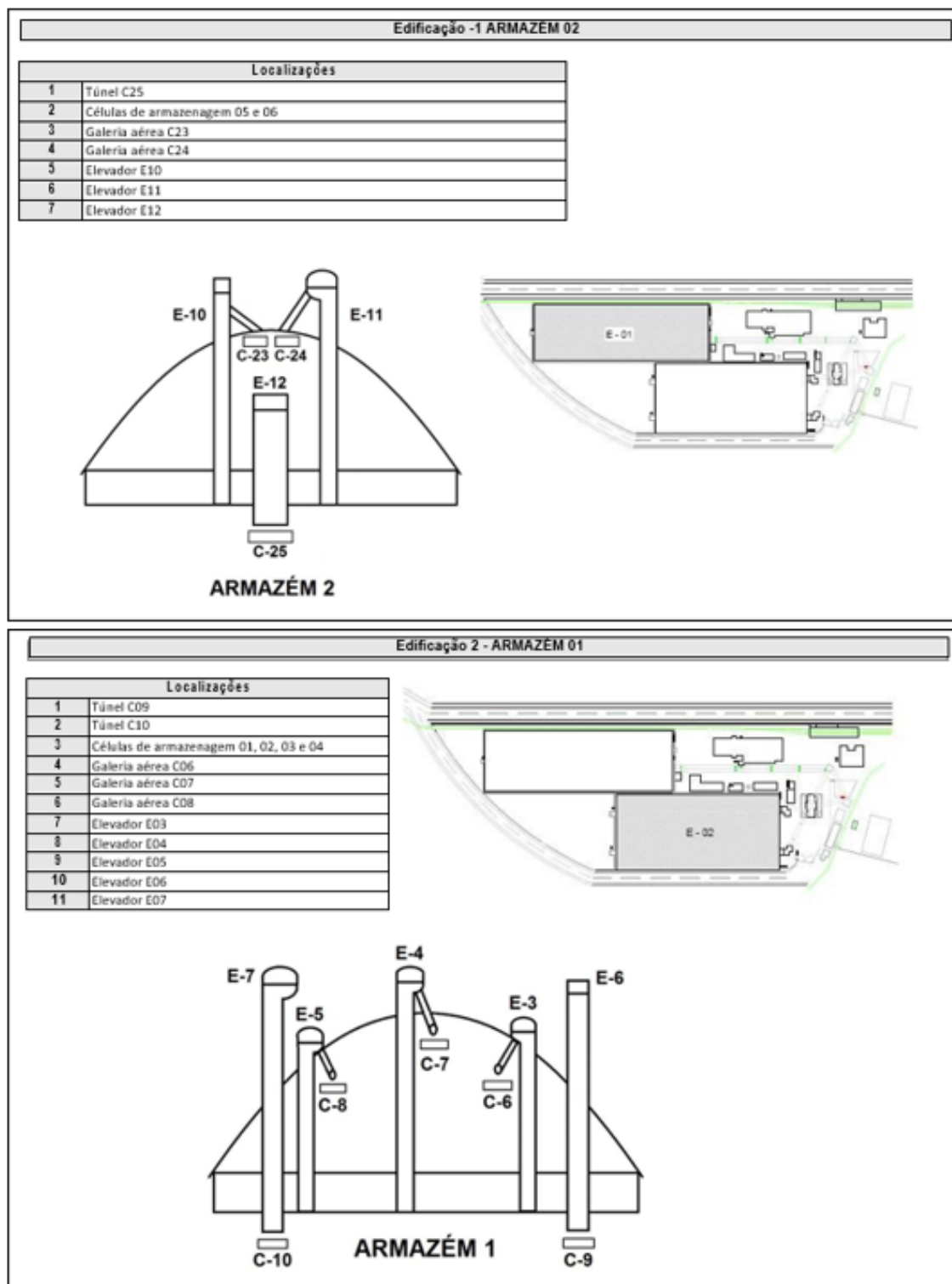
Figura 4 – Armazéns 1 e 2.
