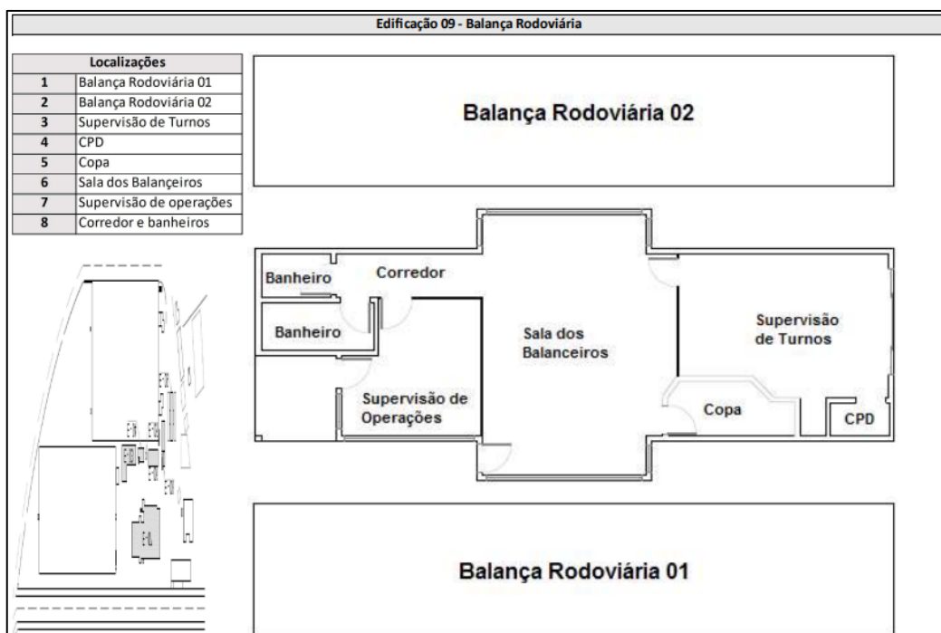
Figura 8 – Balança Rodoviária.
