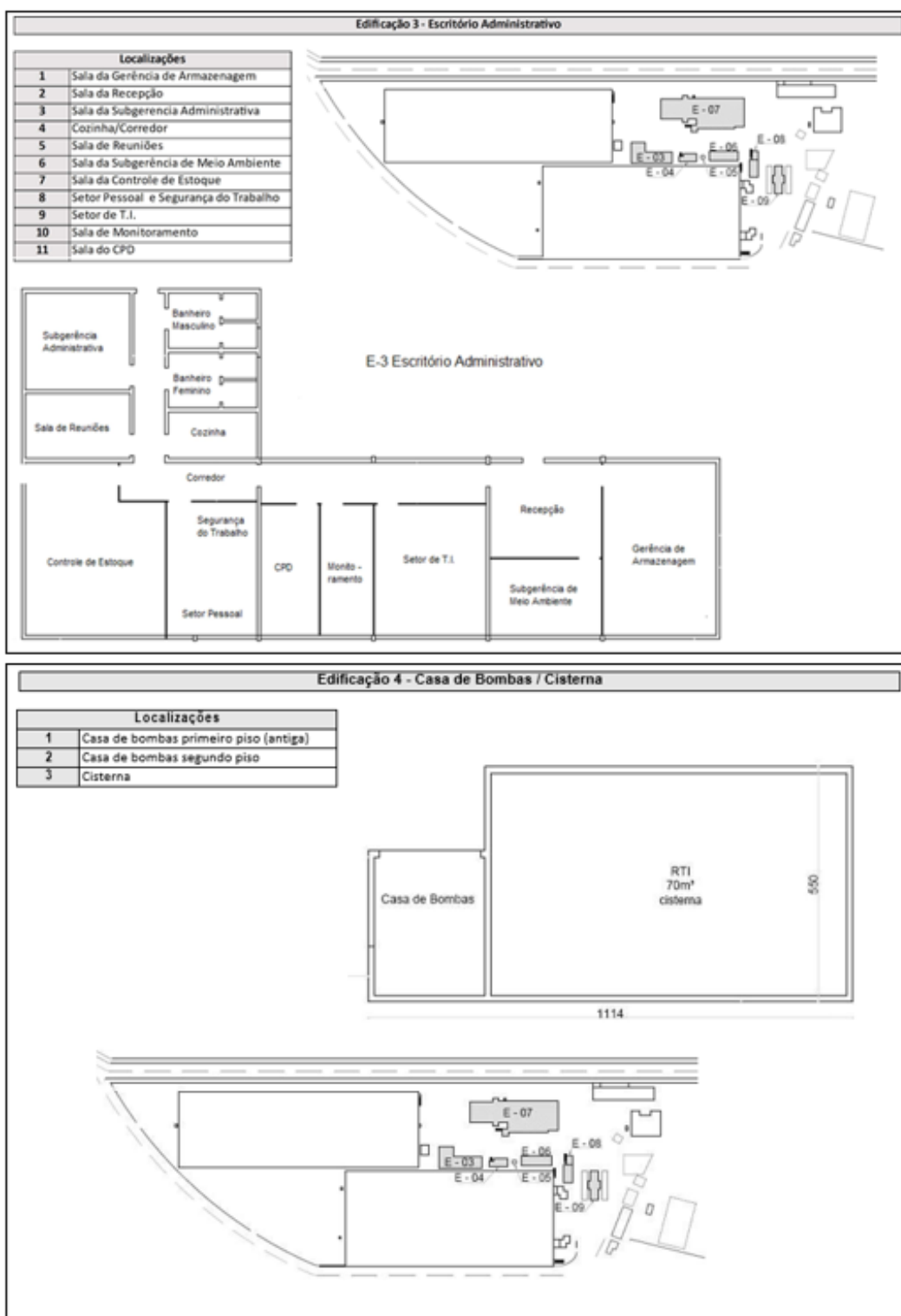
Figura 5 – Escritório administrativo e casa de bombas.
